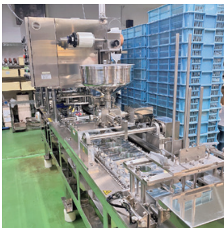
省エネ補助金を活用して導入した清水白桃ゼリー製造機
